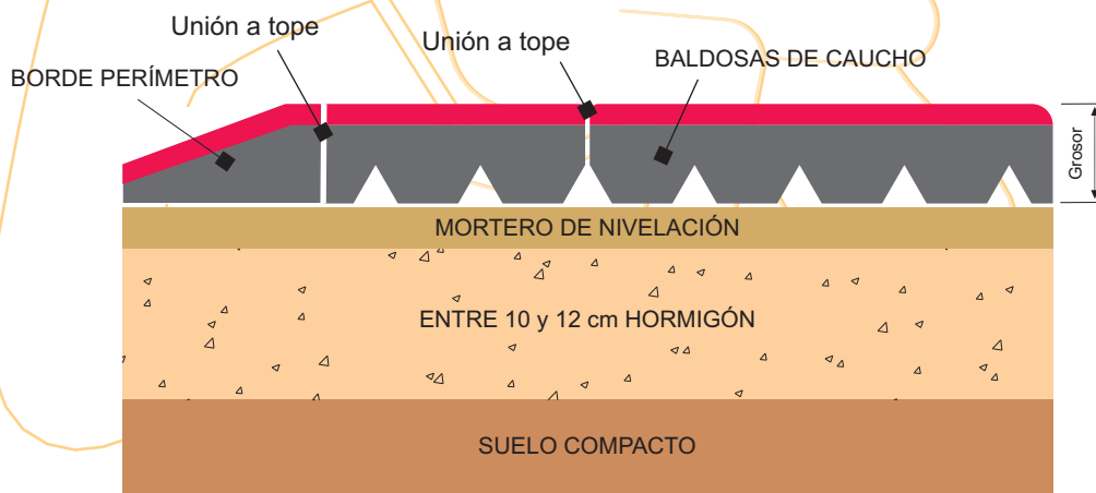
DETALLE DE LA INSTALACIÓN SOBRE BASE DE HORMIGÓN
