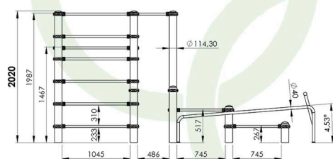
DIMENSIONES GENERALES/ DIMENSIONS GÉNÉRALES/SIMPLE DIMENSIONS
