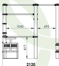
DIMENSIONES GENERALES/ DIMENSIONS GÉNÉRALES/SIMPLE DIMENSIONS
